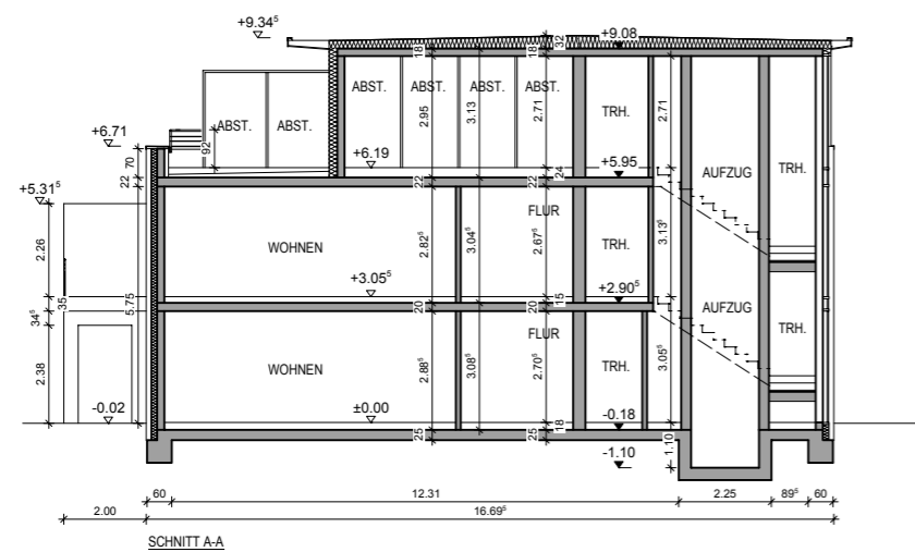
SCHNITT A-A
